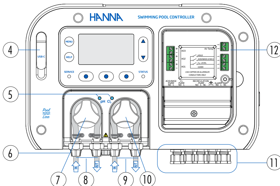
BL131 vista frontal – conectores eléctricos de bajo voltaje expuestos
